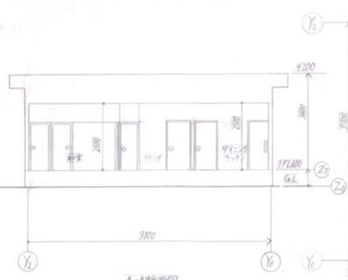
A-立面図
