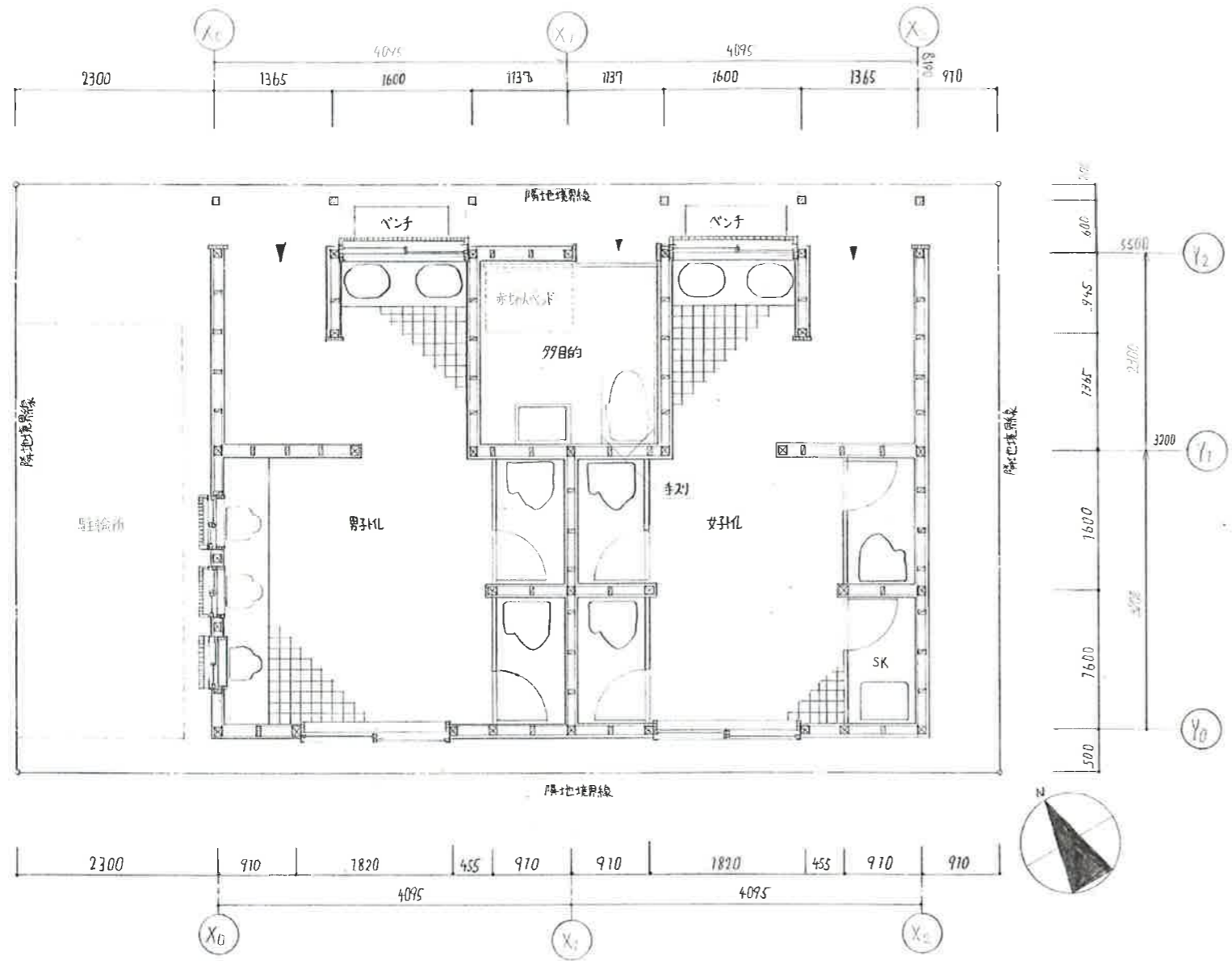
平面図兼配置図 1:50
