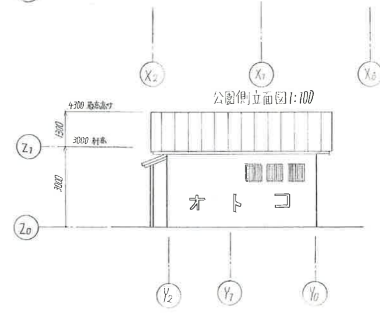
男子側立面図 1:100
