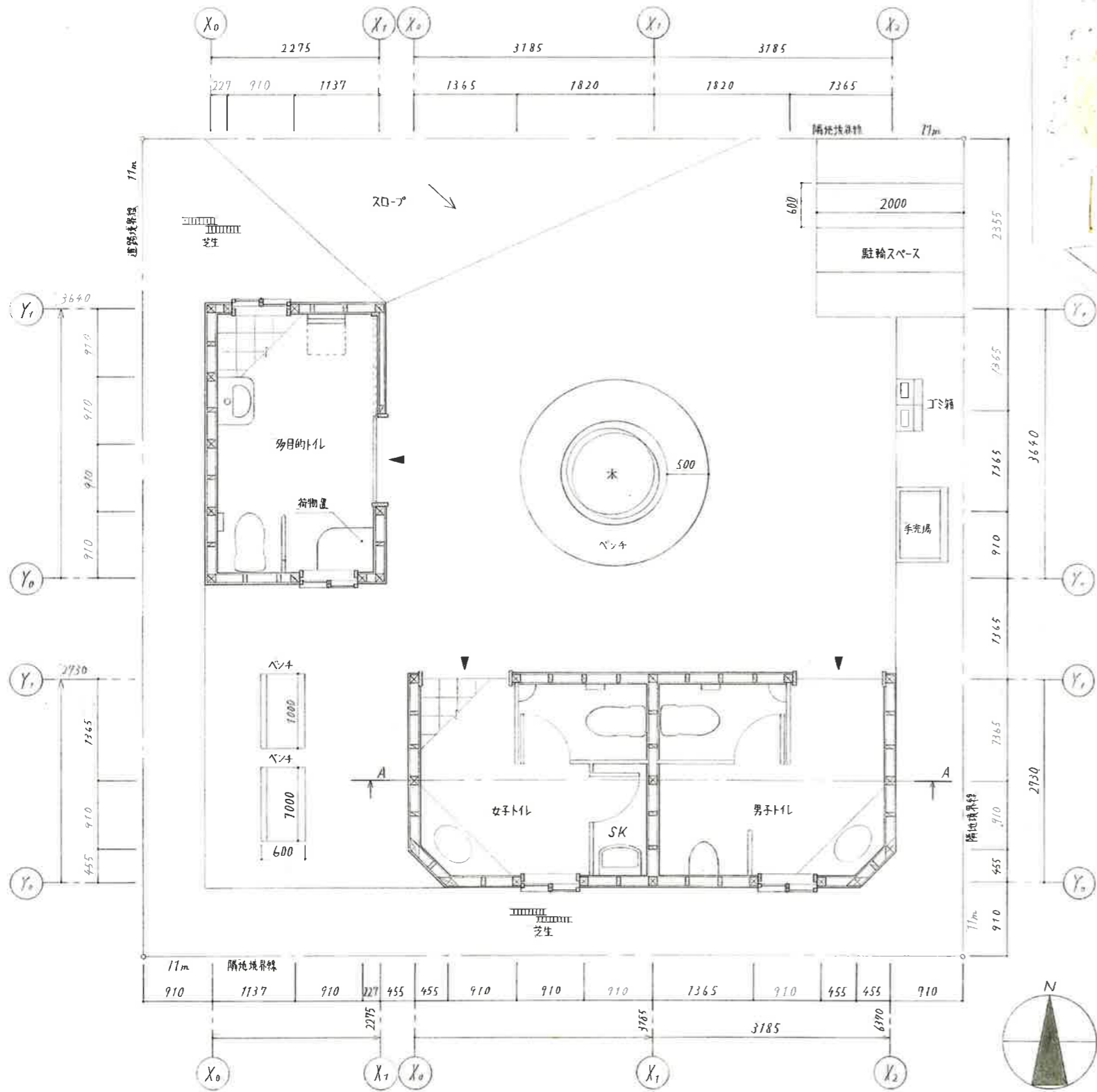
平面図兼配置図 1:50
