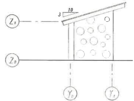
東立面図 1:100
