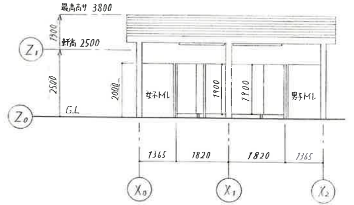
A-A断面図 1:100
