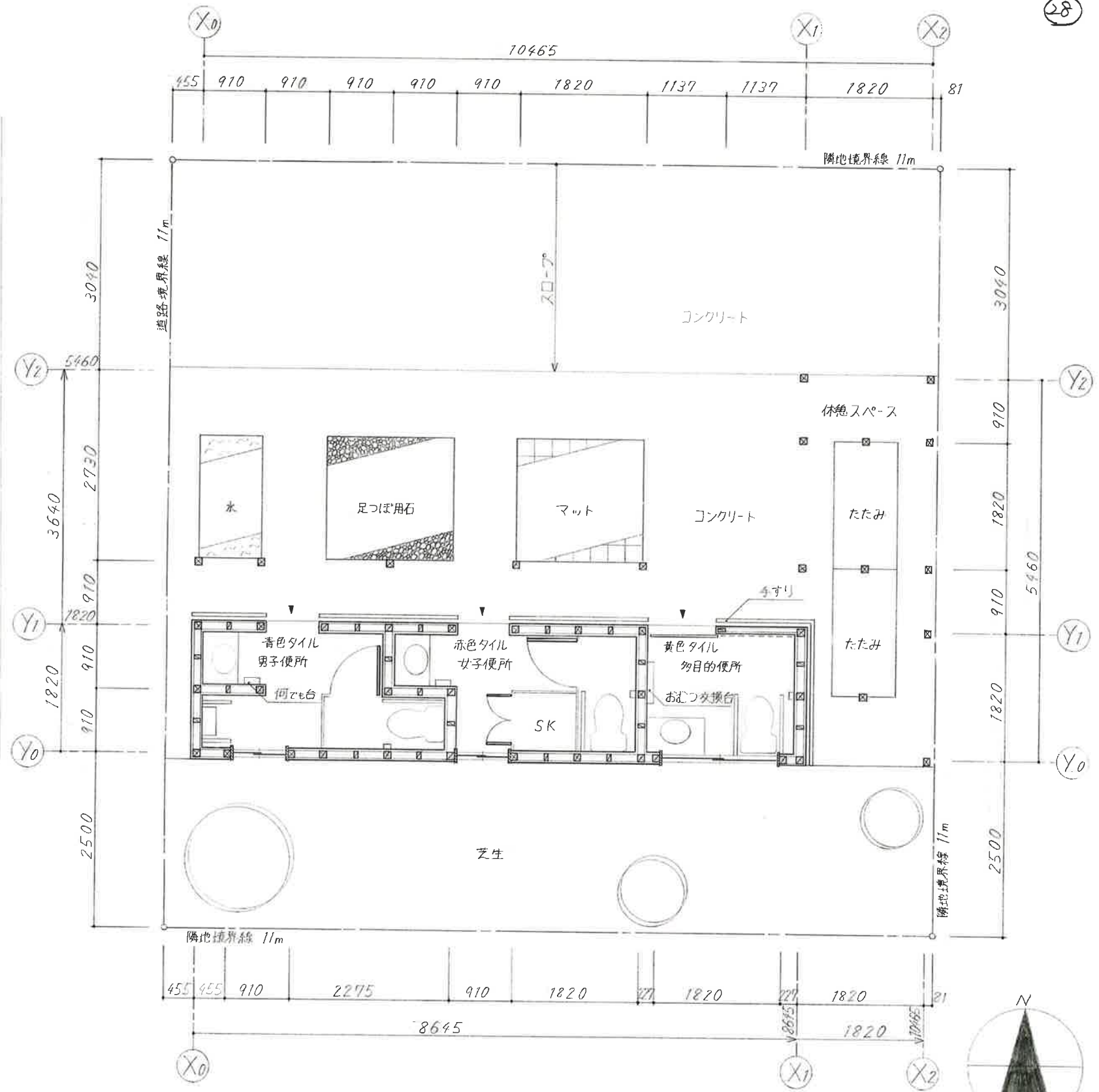
配置図兼平面図 1:50
