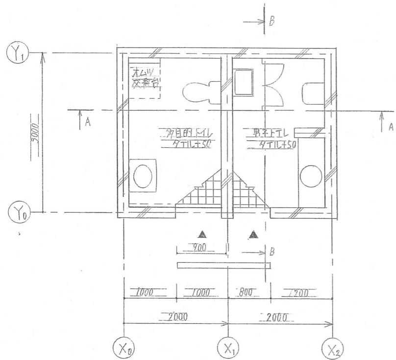
平面図 1:50
