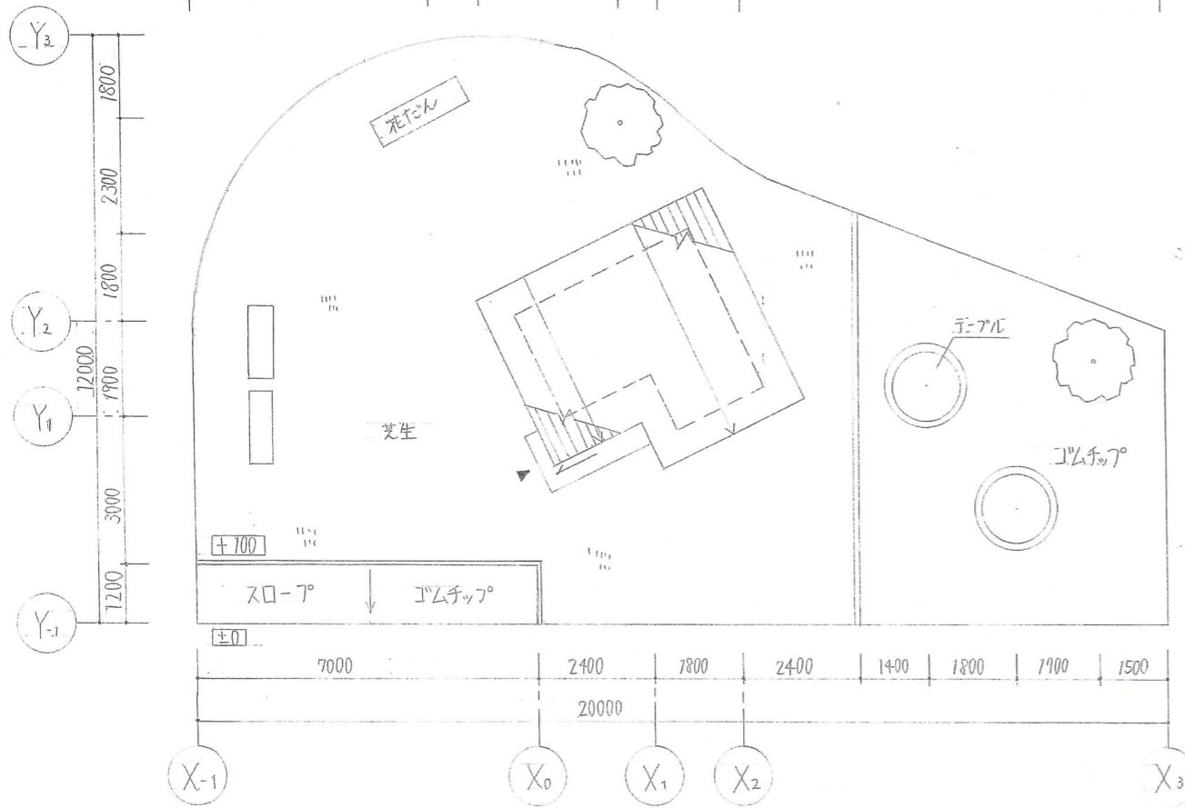
配置図兼屋根状せ図
