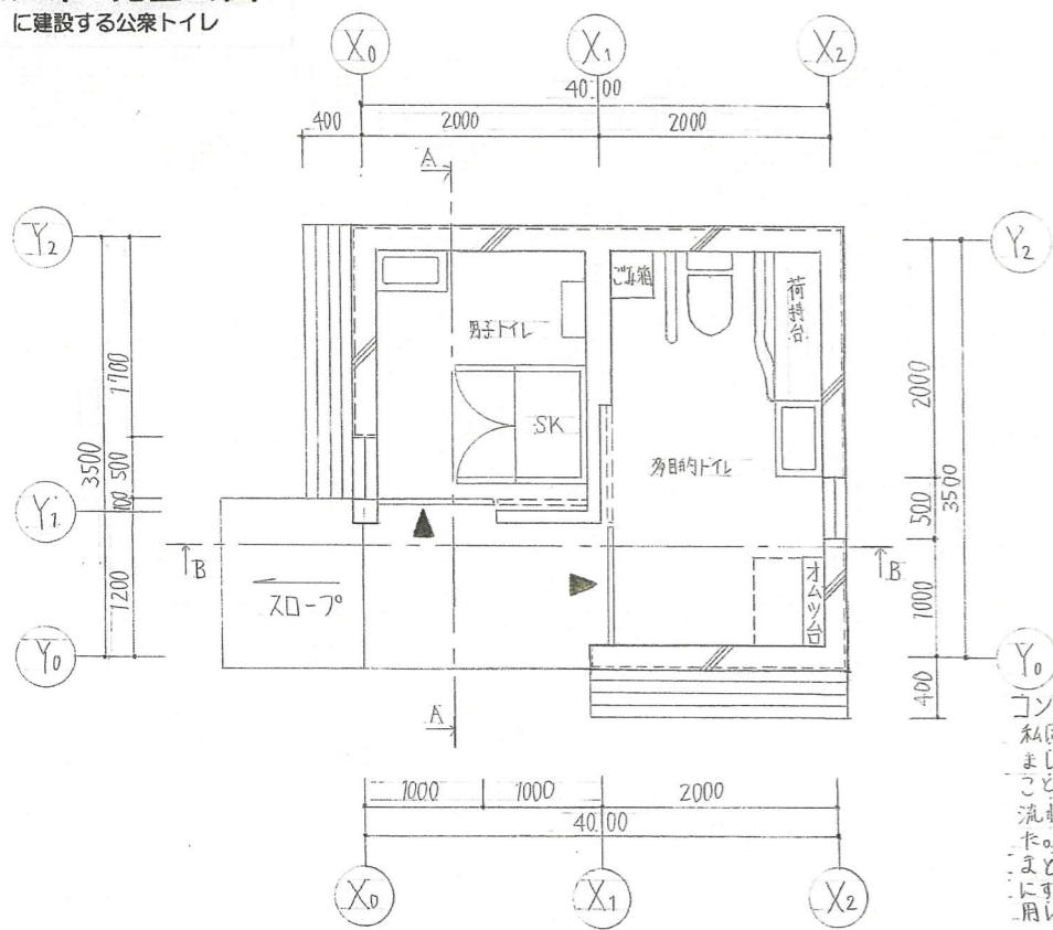
平面図 1:50
