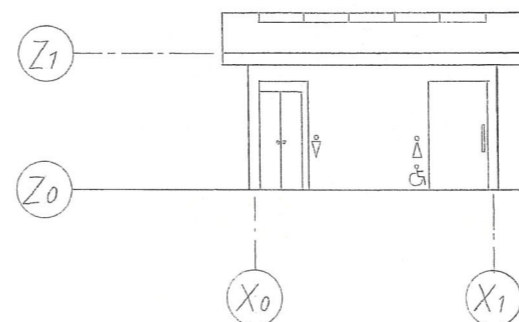
北立面図 1:100
