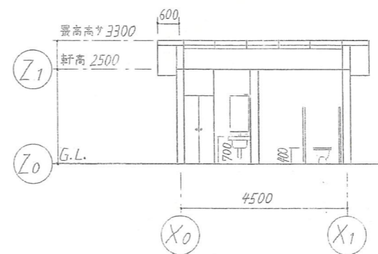
A-A断面図 1:100
