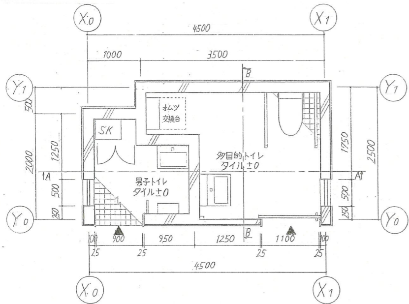
平面図 1:50
