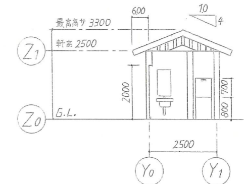
B-B断面図 1:100
